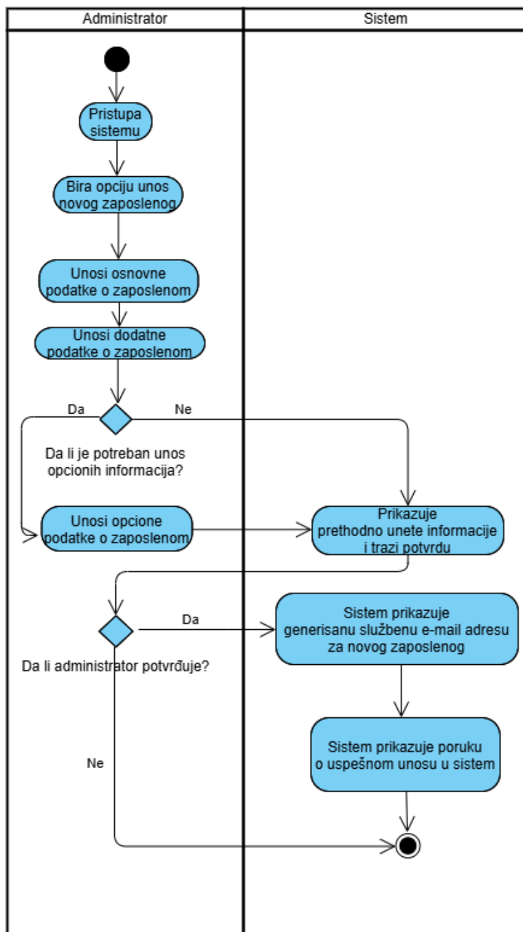
Slika 15: Dijagram aktivnosti "Unos novog zaposlenog"
